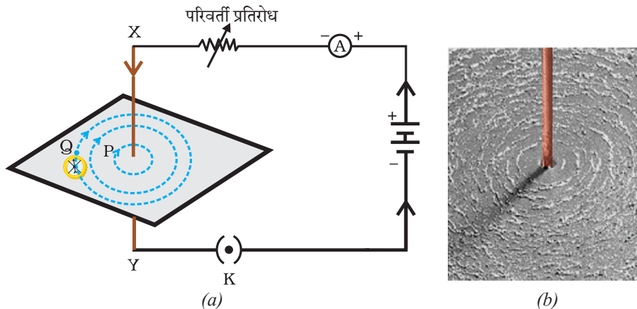
चित्र 12.6 (a) किसी विद्युत धारावाही सीधे चालक तार के चारों ओर के चुंबकीय क्षेत्र की क्षेत्र रेखाओं को निरूपित करता संकेंद्री वृत्तों का पैटर्न। वृत्तों पर अंकित तीर क्षेत्र रेखाओं की दिशाओं को दर्शाते हैं। (b) प्राप्त पैटर्न का समीप दृश्य
