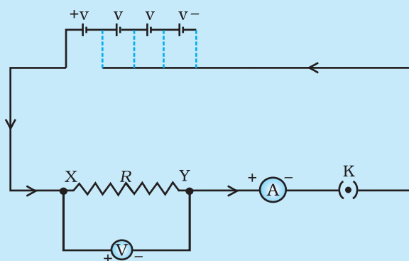
चित्र 11.2 ओह्म के नियम के अध्ययन के लिए विद्युत परिपथ
