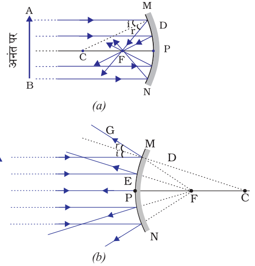
चित्र 9.2 (a) अवतल दर्पण (b) उत्तल दर्पण
