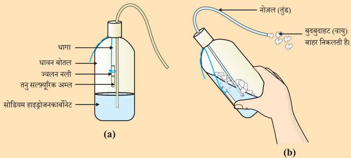
चित्र 2.10 (a) सोडियम हाइड्रोजनकार्बोनेट वाली धावन बोतल में लटकी हुई तनु सल्फ्यूरिक अम्ल वाली ज्वलन नली (b) नोजल से बाहर आती बुदबुदाहट
